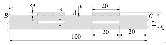
图 9 磁电弹传感器(单位:mm) Fig.9 Magneto-electro-elastic sensor(unit:mm)
