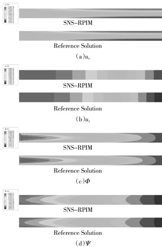
图 7 悬臂梁 u_x 、 u_z 、 \Phi 和 \Psi 云图 Fig.7 Contour of u_x 、 u_z 、 \Phi and \Psi of cantilever beam
