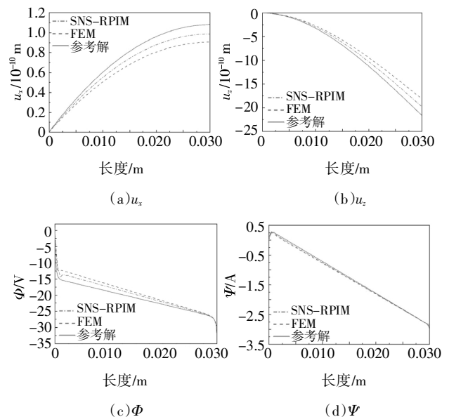
图6 悬臂梁AB边界处 u_x, u_z, \Phi 和 \Psi 变化趋势
