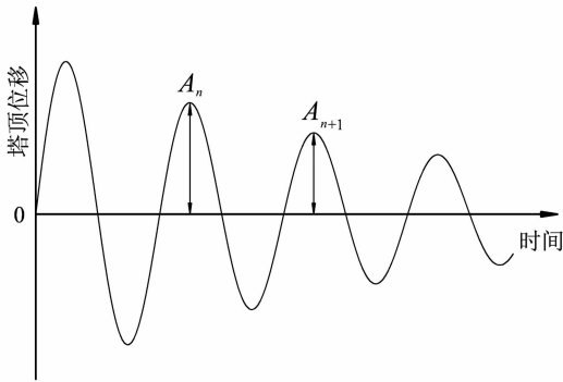
图 2 塔顶振动衰减示意图
