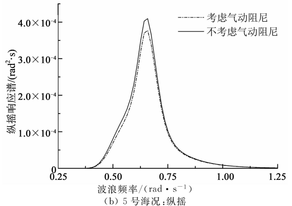
图5 第5号海况中考虑与不考虑气动阻尼响应谱对比
