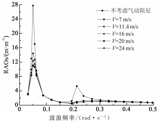
(a) 作业工况: 纵荡
