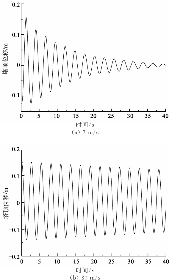
图 3 塔顶位移衰减曲线
